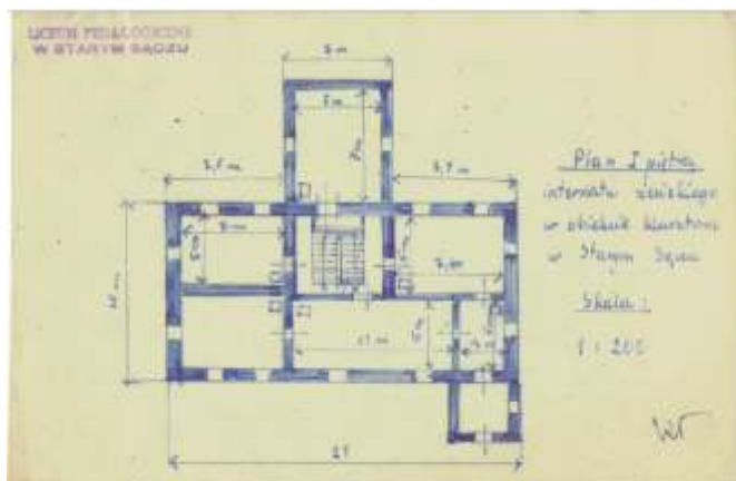
Plan I piętra dawnego Internatu Liceum Pedagogicznego w budynkach klasztornych (Archiwum Internatu)
